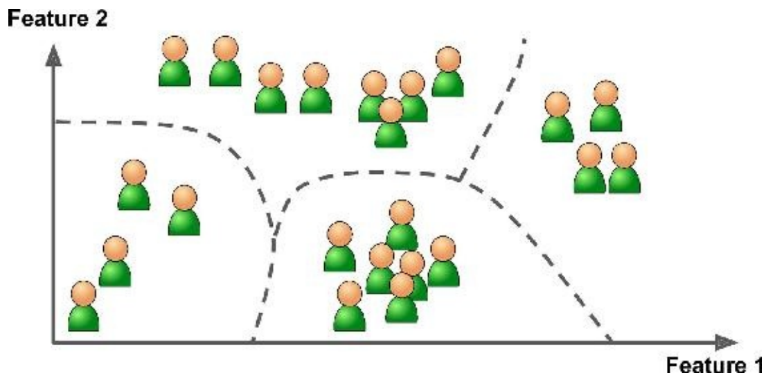
Figure 1-8. Clustering
